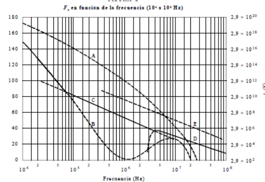
A: Ruido atmosférico, valor excedido durante el 0,5% del tiempo B: Ruido atmosférico, valor excedido durante el 99,5% del tiempo C: Ruido artificial, punto de recepción tranquilo D: Ruido galactico E: Ruido artificial mediano en una zona comercial
