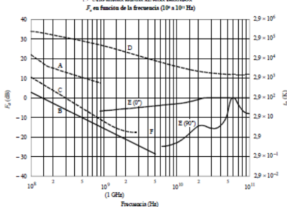
A: Ruido artificial mediano en una zona comercial B: Ruido galactico C: Ruido galactico (en direccion del centro galactico para un haz infinitamente estrecho) D: Sol en calma (haz con 1/2 grado de abertura orientado hacia el Sol) E: Ruido del cielo debido al oxigeno y al vapor de agua (nubes de haz muy estrecho); curva superior, ángulo de elevación 0°, curva inferior, ángulo de elevación 90° F: Cuerpo negro (ruido de fondo cósmico), 2,7 K
